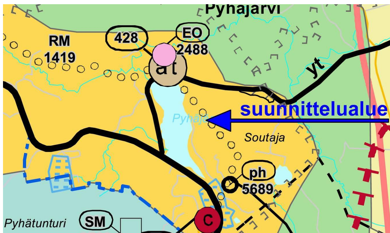
Kuva 5. Rovaniemi-Itä-Lapin maakuntakaavaehdotus 25.4.2022.
